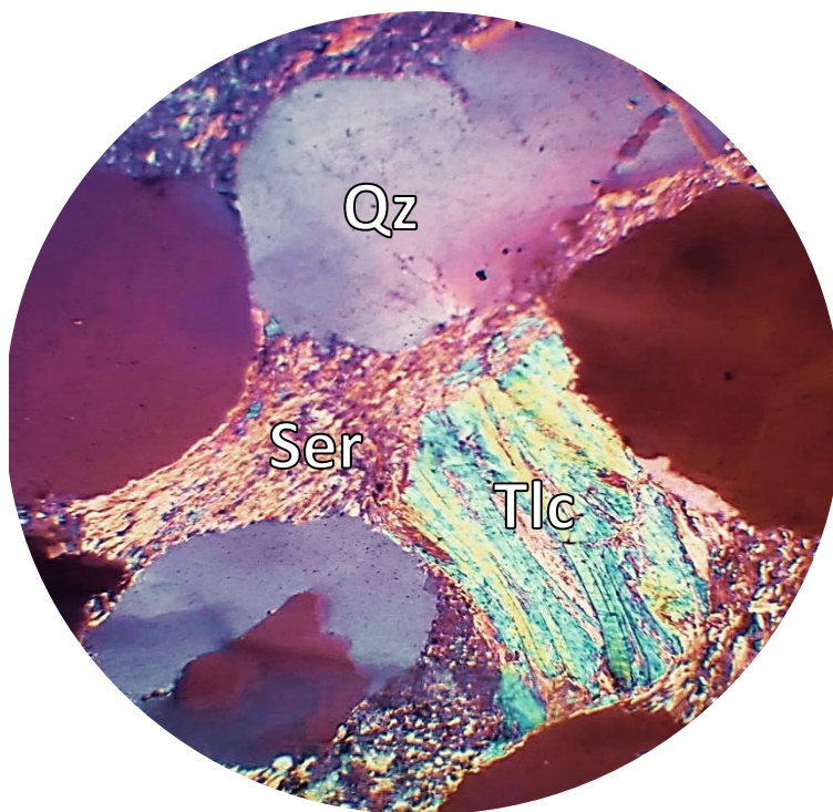
Рис.4.7 - Кварцит зі слюдистим цементом та уламком розщепленого талькового сланцю (аналог «гнучкого» алмазовміщуючого сланцю ітаколуміту району Діамантіна, Бразилія). Шліф, нік +, зб.90.
