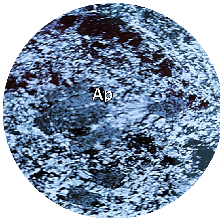
Рисунок 4.8 – Порфірові агрегати апатиту з проявами катаклазу та субпаралельною орієнтовкою порфірових вкраплень.
