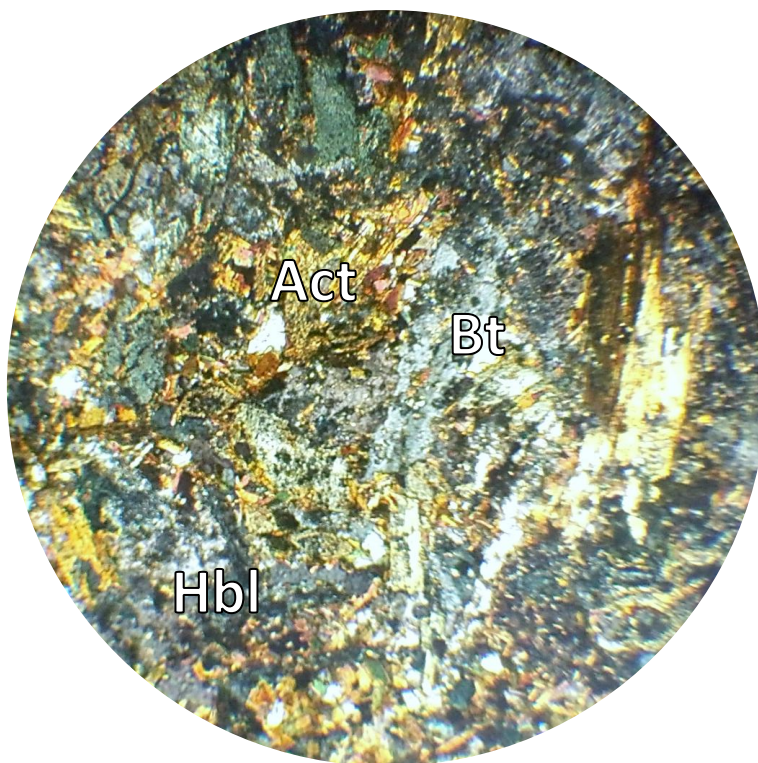
Рисунок 3.5 – Апобазальтовий амфіболіт, біотитизований.
