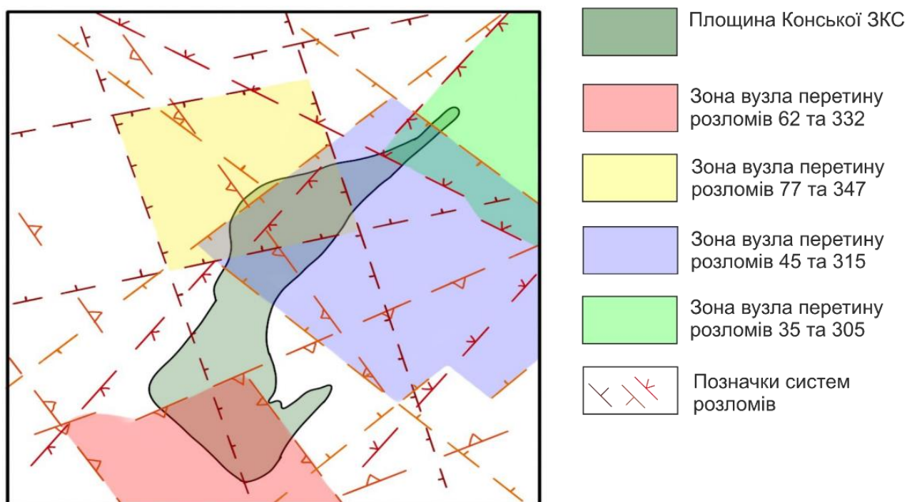
Рисунок 3.31 – Розташування Конкської ЗКС у вузлі перетину систем глибинних розломів Середньпридніпровського мегаблоку.
