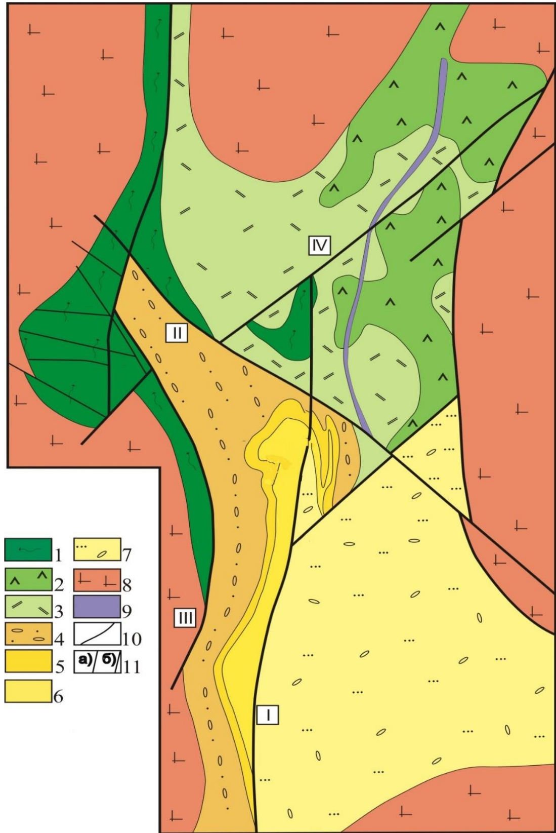
Рисунок 3.1 – Схема геологічної будови Білозерської структури за даними УкрДГРІ, 2006 [90]. Умовні позначення на стор.35
