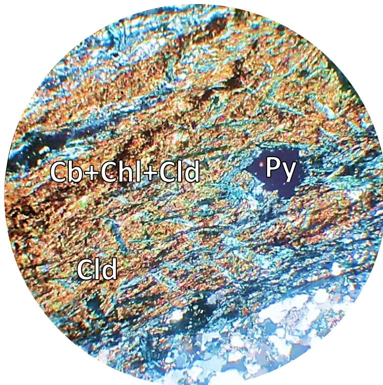
Рисунок 3.9 – Філіт кварц-карбонат-хлорит-хлоритоїд-серицитовий з мінералізацією піриту. Нік+, зб.90
