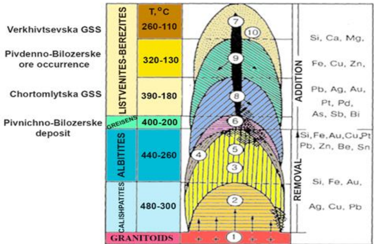
Рисунок 4.15 – Розташування зон метасоматитів, що вміщують зруденіння дорогоцінних металів у межах ЗКС Середньопридніпровського мегаблоку в схемі О.Ф.Коробейнікова [116]
