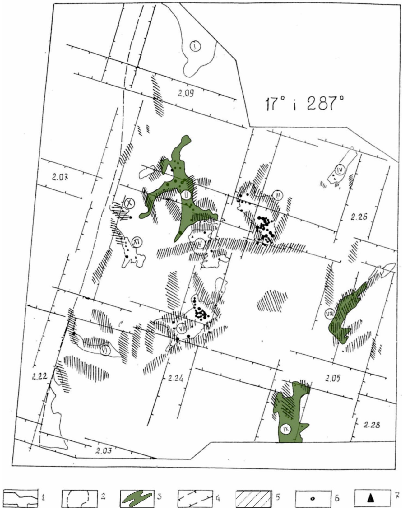
Рисунок 3.34 – Розташування золоторудних проявів, ділянок метосоматозу та зеленокам'яних структур відносно системи розломів з азимутами простягання 17° і 287° (Умовні позначення на стор. 91)
