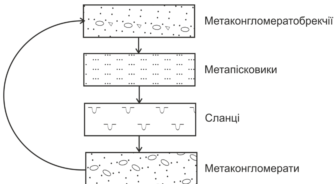
Рисунок 3.19 – Схема градаційної шаруватості
