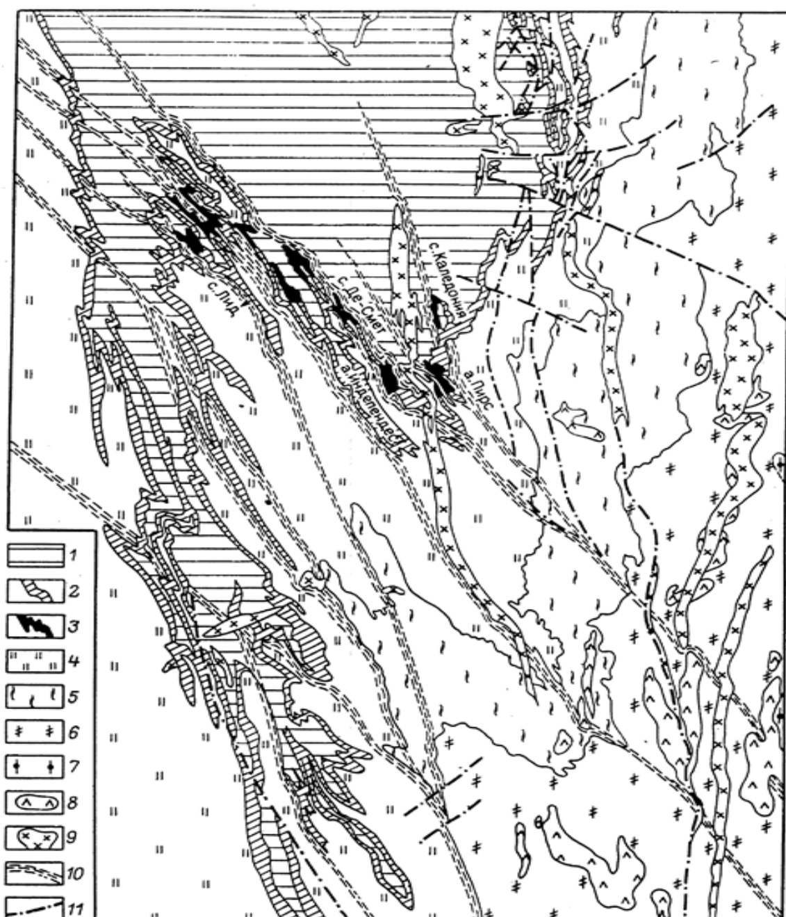
Рисунок 4.14– Геологічна схема рудного поля Хомстейк. За матеріалами К. Конді [34]
