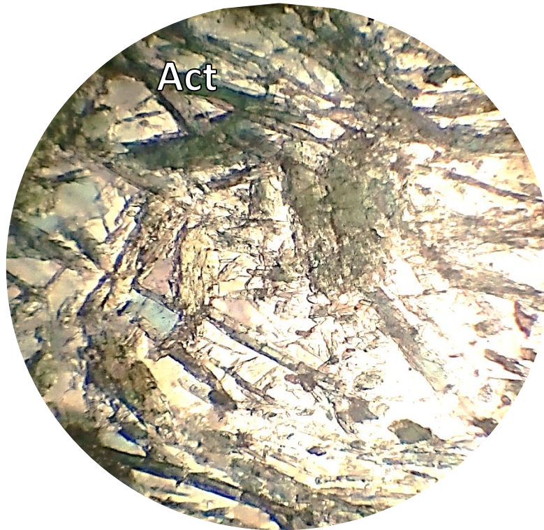
Рис. 3.30 – Метакоматіт гломеробластової структури, з реліктами структури «спініфлекс» олівин-піроксенового типу. Св.1355
