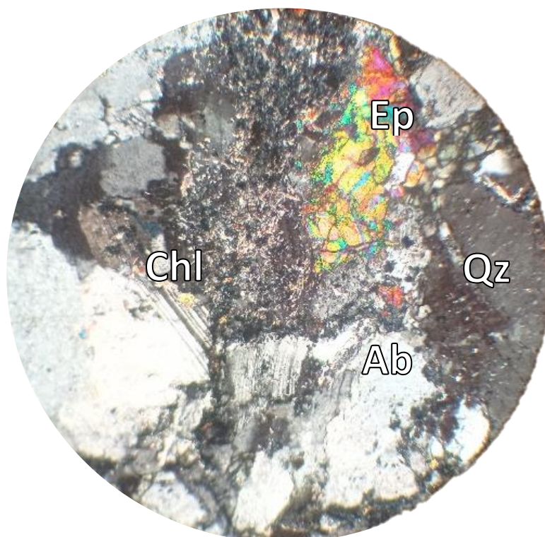
Рисунок 4.17 - Хлорит-карбонат-епідот-кварц-альбітовий метасоматит.
