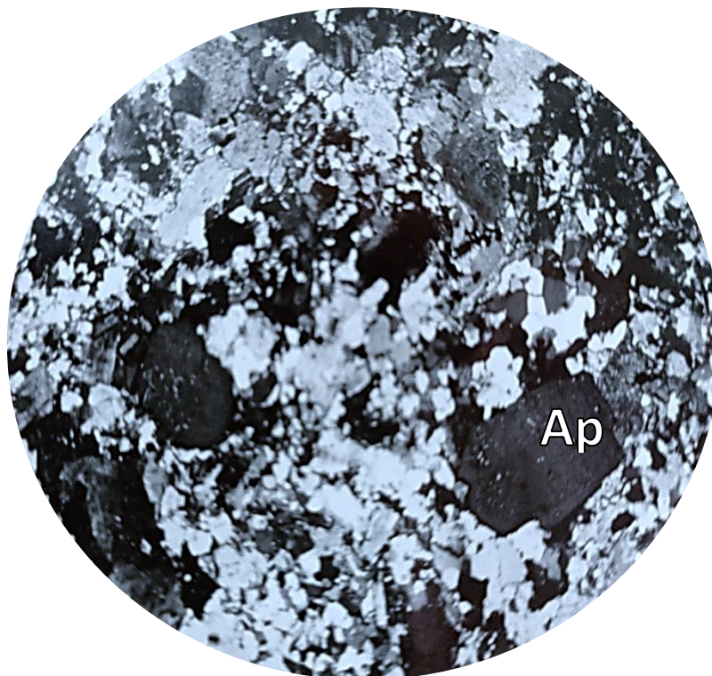
Рисунок 4.9 – Порфіроподібні агрегати апатиту в дрібнозернистій катаклазованій біотит-плагіоклаз-мікрокліновій масі.
