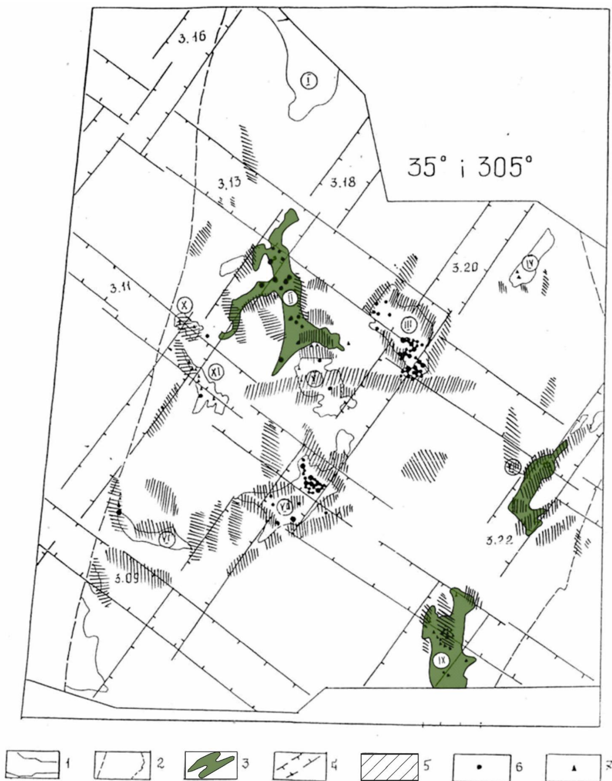
Рисунок 3.35 – Розташування золоторудних проявів, ділянок метосоматозу та зеленокам'яних структур відносно системи розломів з азимутами простягання 35° і 305°
