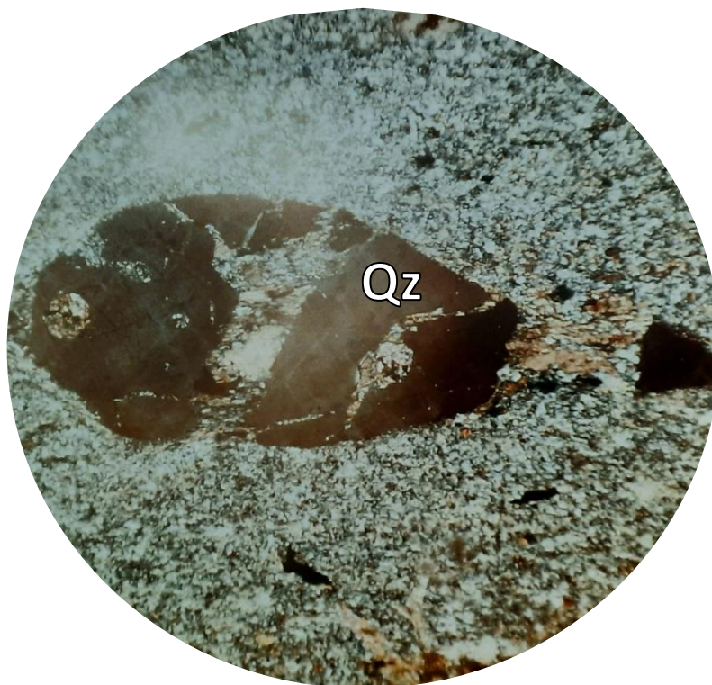
Рис.4.4 — Структура «in situ» (підірваних на місці ксенолітів) уламку кварцу та флюїдальність серицитових агрегатів з корозією кварцевих зерен.
