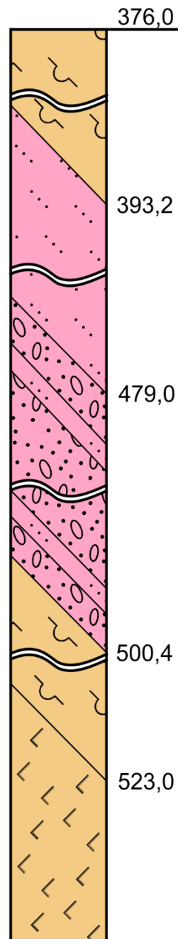
Рисунок 3.17 - Геологічна колонка по свердловині №507
