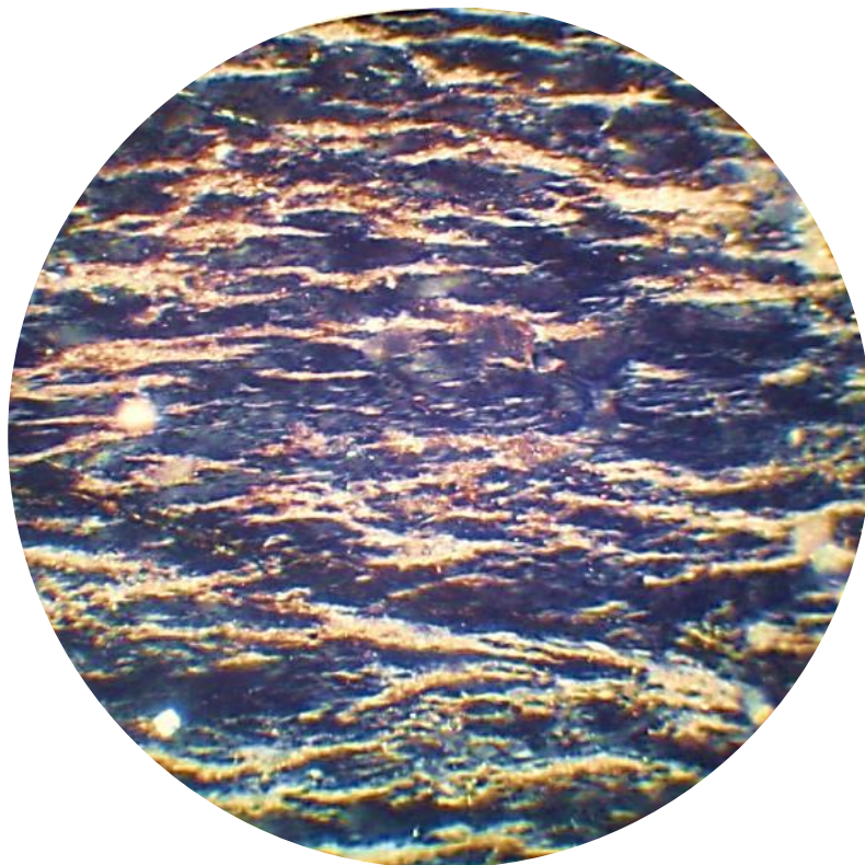
Рис.4.3– Флюїдальна мікротекстура карбонатної речовини флюїдоліту тимошівської товщі. Шліф, нік+, зб.104
