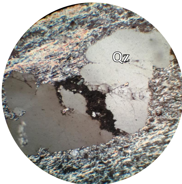
Рисунок 3.23 – Структура «in situ» у зерен кварцу. Кородування зерен кварцу кварц-серицитовою речовиною.
