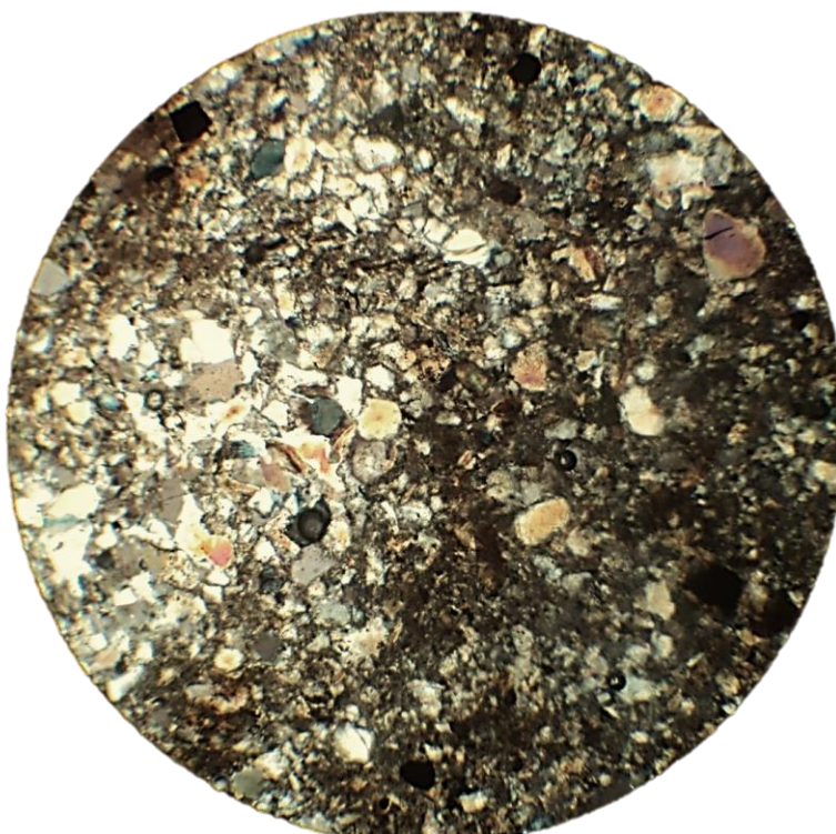
Рисунок 3.11 – Метаалевроліт аркозовий михайлівської світи (БЗКС).
