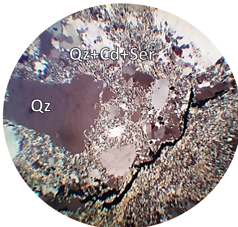
Рисунок 3.22 – Кородування уламків кварцу із заміщенням їх новоутвореними кварц-карбонат-серицитовими агрегатами, регенерація кварцу по контурах окремих уламків, розвиток піриту по тріщині в цементі метаконгломератобрекчії. 36.90, нік+.
