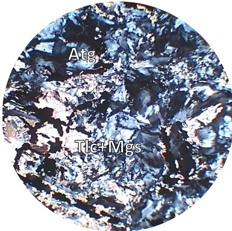
Рисунок 4.18 – Розвиток тальк-магнезитових агрегатів по хризотилу в серпентиніті Варварівського масиву.
