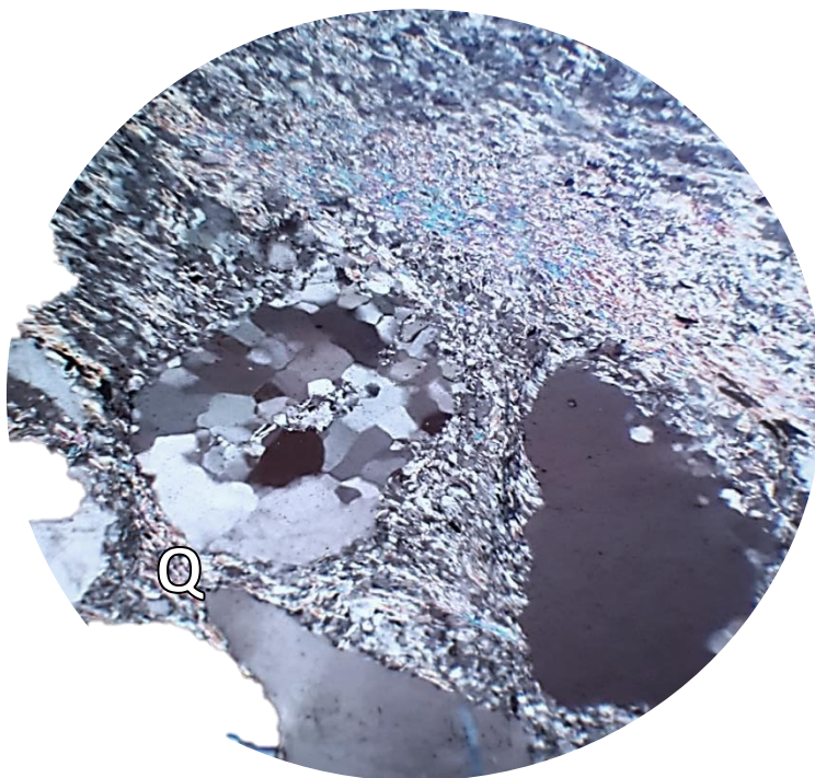
Рис.4.5 – Структура «сніжної грудки» уламків кварциту, уламки обкатаної та незграбної форми, флюїдальність кварц-серицитових агрегатів в цементі метаконгломератобрекчії.
