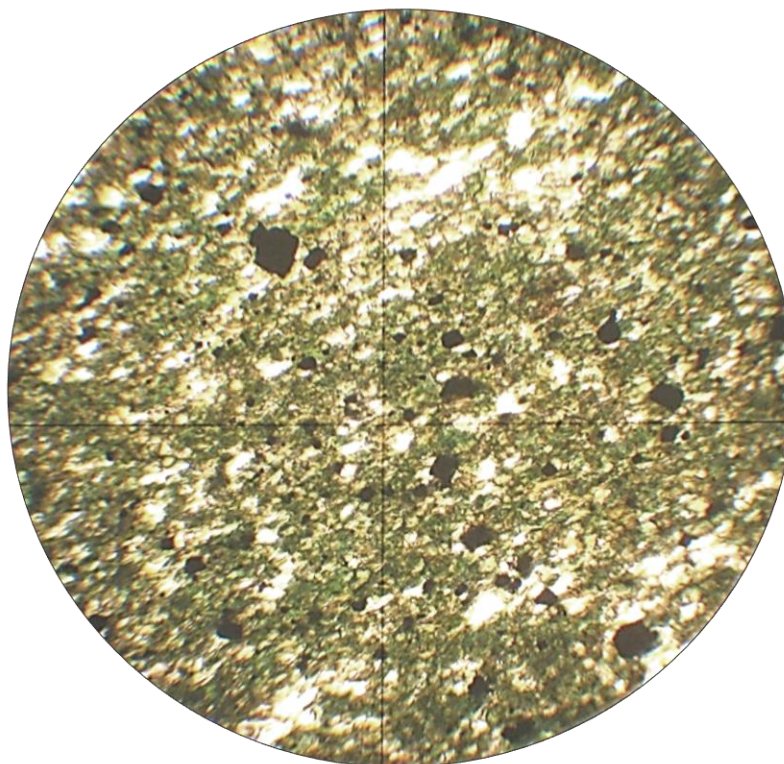
Рисунок 3.7 - Кварц-біотит-- серицит-карбонат-хлоритовий сланець з вкрапленістю сульфідів. Шліф, Ніколі II, зб. 90 ×.
