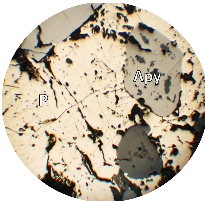
Рисунок 4.10 – Рудна мінералізація халькопірит-піритового складу колчеданних прошарків магнетит-хлоритових сланців білозерської серії.
