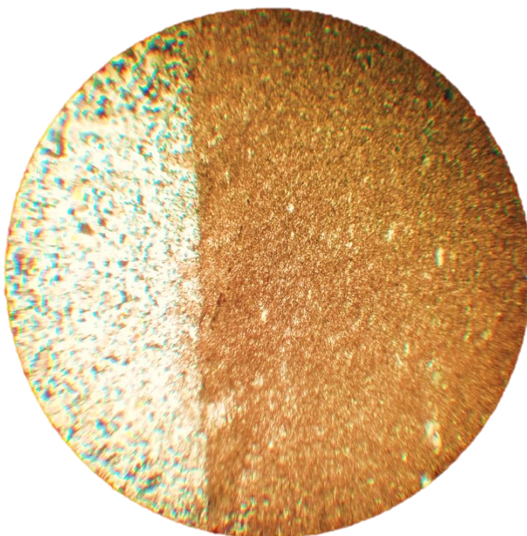
Рисунок 3.12 – Кварцевий сидеритоліт (михайлівська світа, БЗКС)
