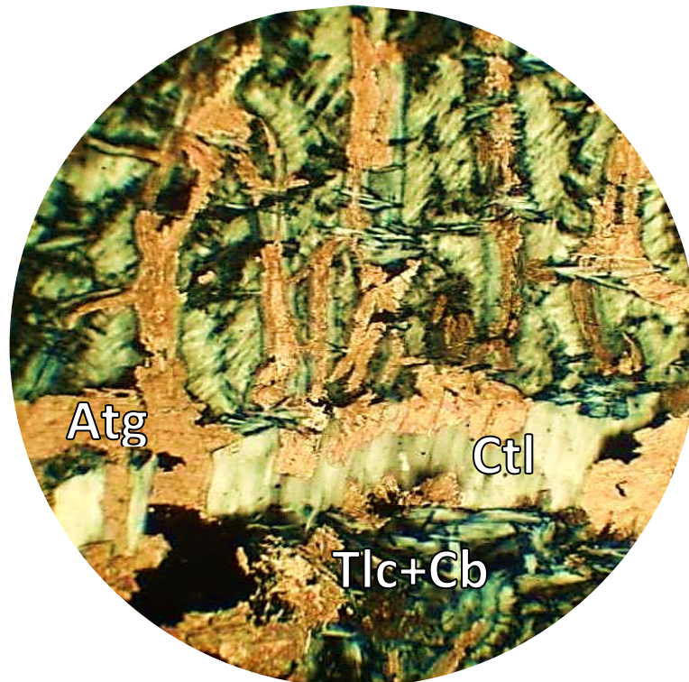
Рисунок 3.3 – Розвиток тальк-карбонатних агрегатів по антигориту та хризотилу в серпентиніті (БЗКС)
