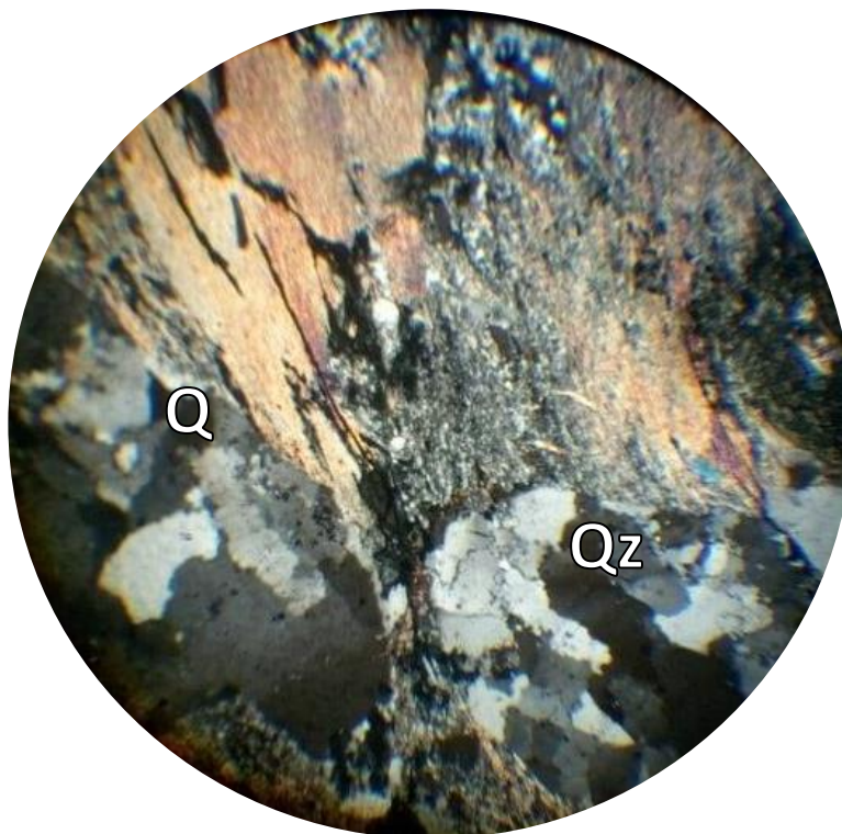
Рисунок 3.13 – Уламки кварцу та безрудного кварциту, агрегати новоутвореного біотиту, заміщення цементу новоутвореними карбонат-серицитовими агрегатами з флюїдальною мікротекстурою.
