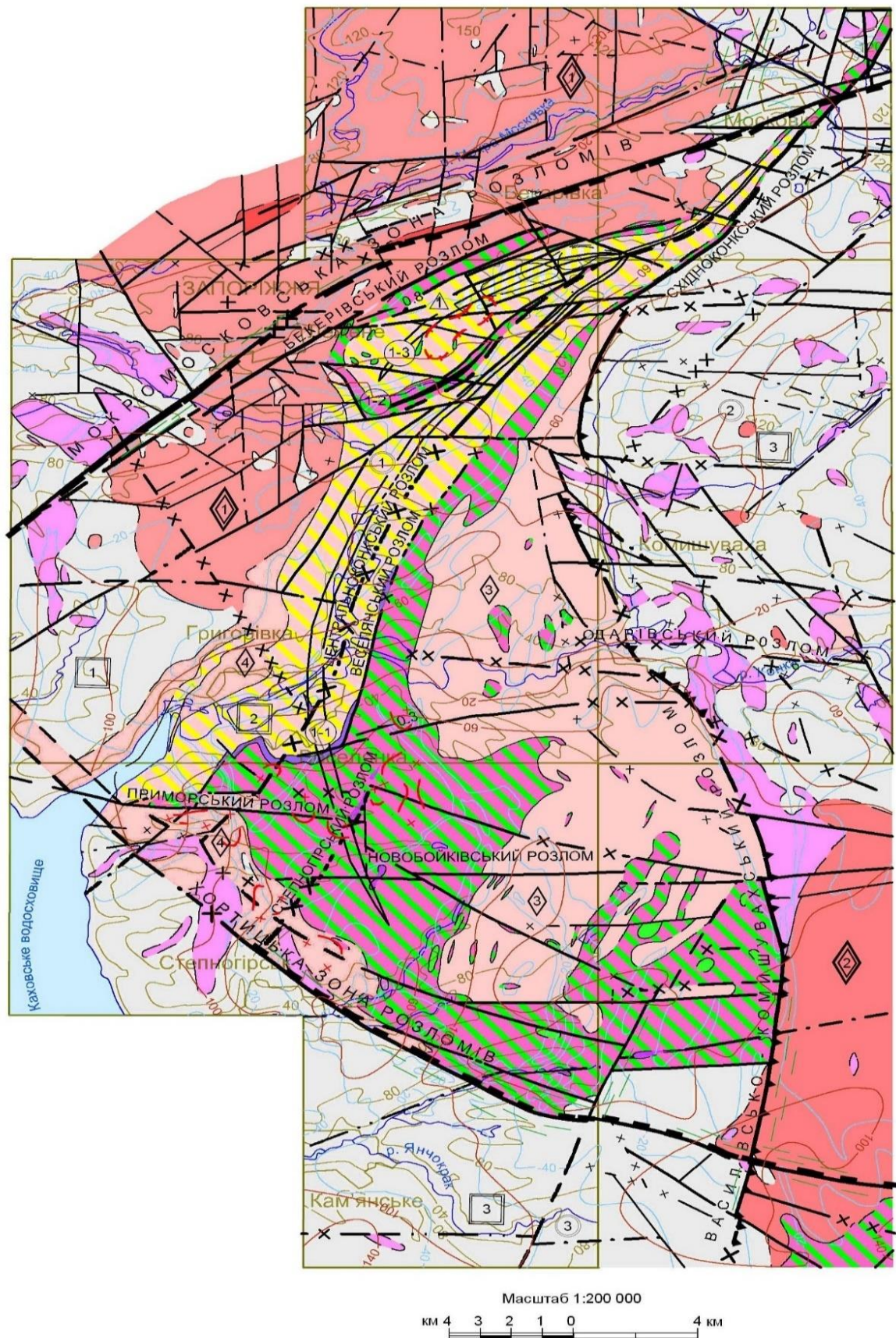
Рисунок – 3.28 - Тектонічна схема кристалічного фундаменту Конкської структури [7] (Умовні позначення на рис. 3.29)
