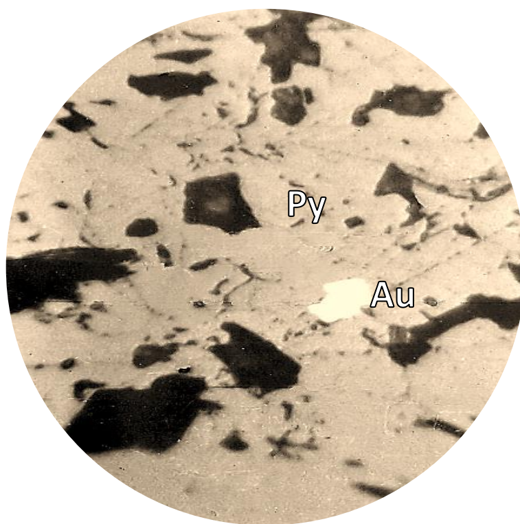
Рисунок 4.13 - Включення самородного золота в піриті. Аншліф, Нік II, зб.500
