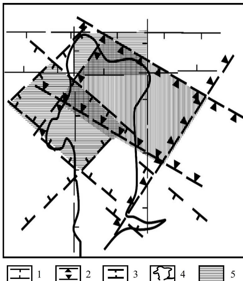
Рисунок 4.11 - Розташування Білозерської ЗКС у вузлі перетину систем глибинних розломів.
