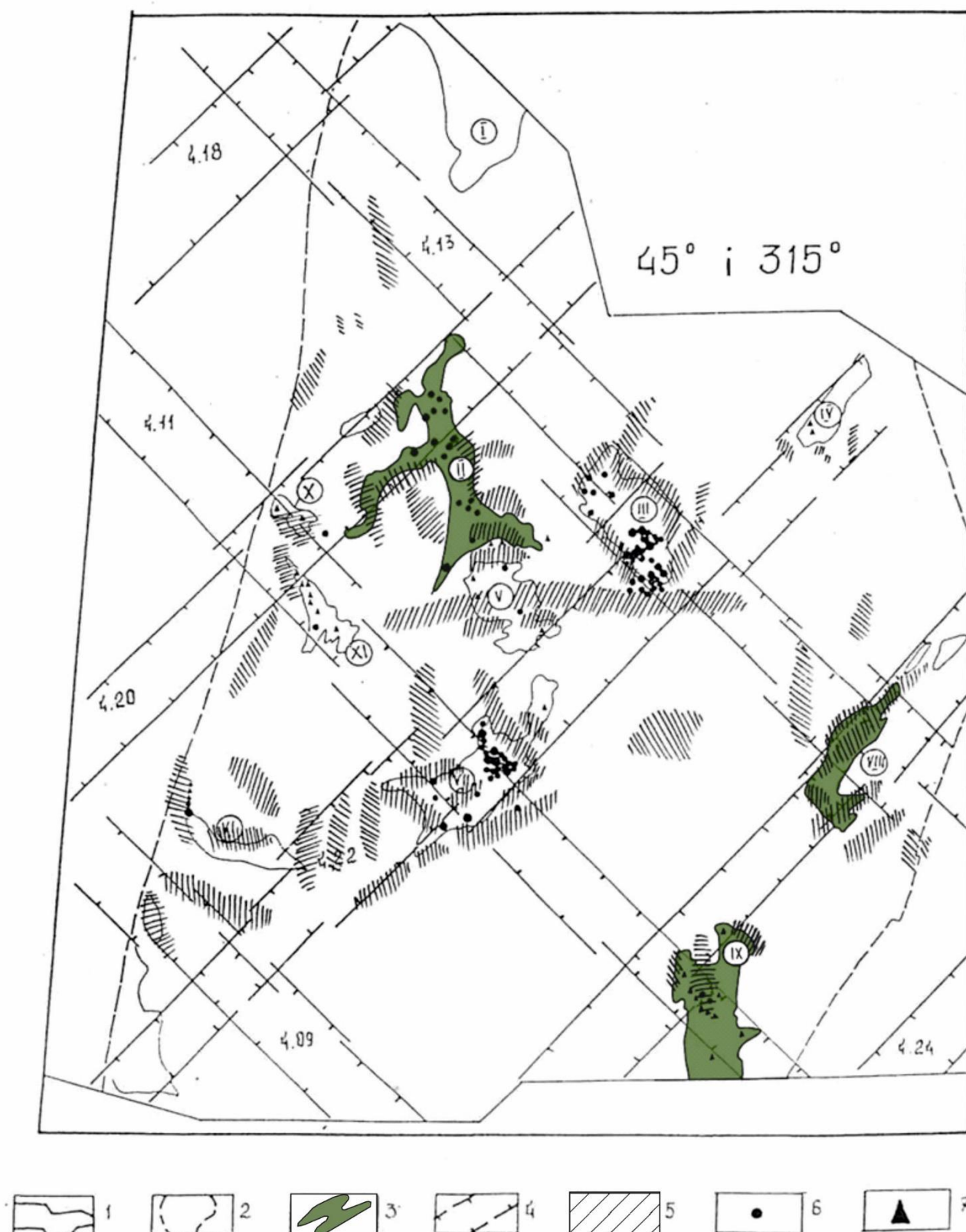
Рисунок 3.36 – Розташування золоторудних проявів, ділянок метасоматозу та зеленокам'яних структур відносно системи розломів з азимутами ліній простягання 45° і 315° (Умовні позначення на стор. 92)
