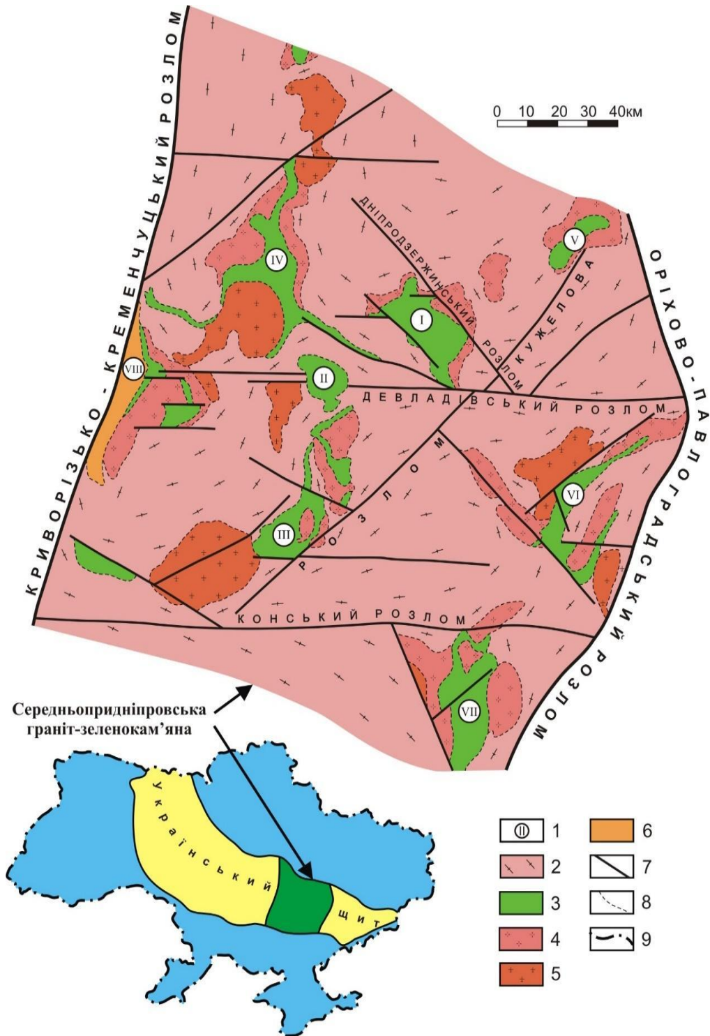
Рисунок 1.1 - Геологічна схема Середнього Придніпров'я за даними УкрДГРІ, 2006 [90]. Умовні позначення на стор.21
