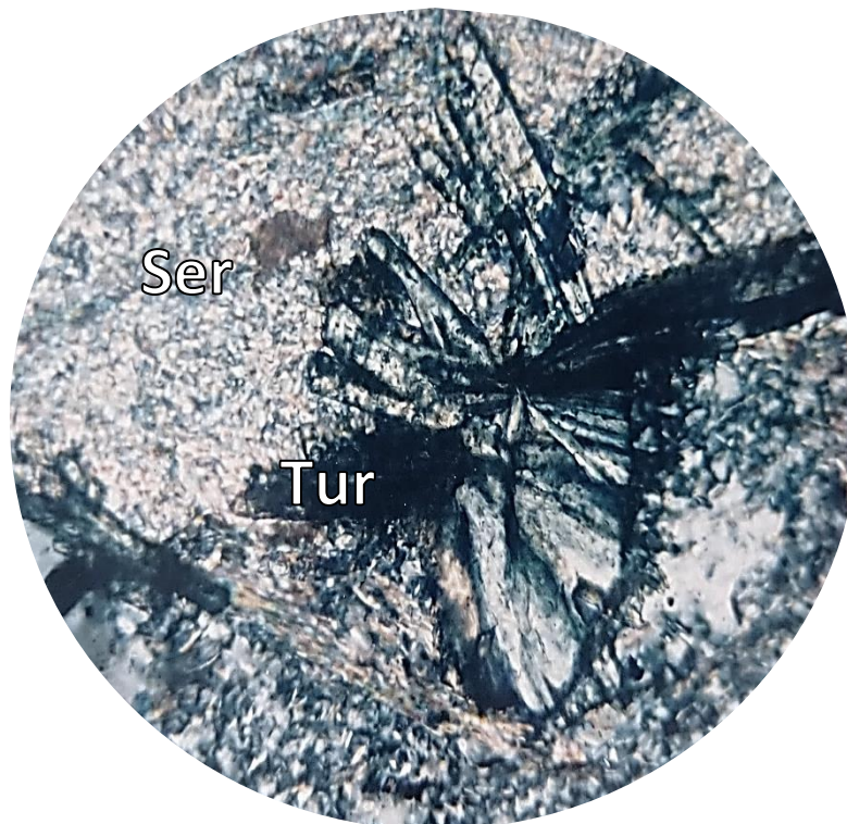
Рисунок 3.24 – «Сонцеподібні» агрегати турмаліну серед серицитових агрегатів в цементі метаконгломератобрекчії.
