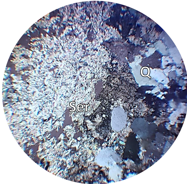
Рисунок 3.21 – Уламки кварциту та серицитизація цементу метаконгломератобрекчії тимошівської товщі.
