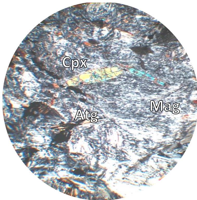
Рисунок 3.4 – Серпентиніт антигоровий з реліктами клінопіроксену та гістерогеним магнетитом по контурах зерен клінопіроксену.
