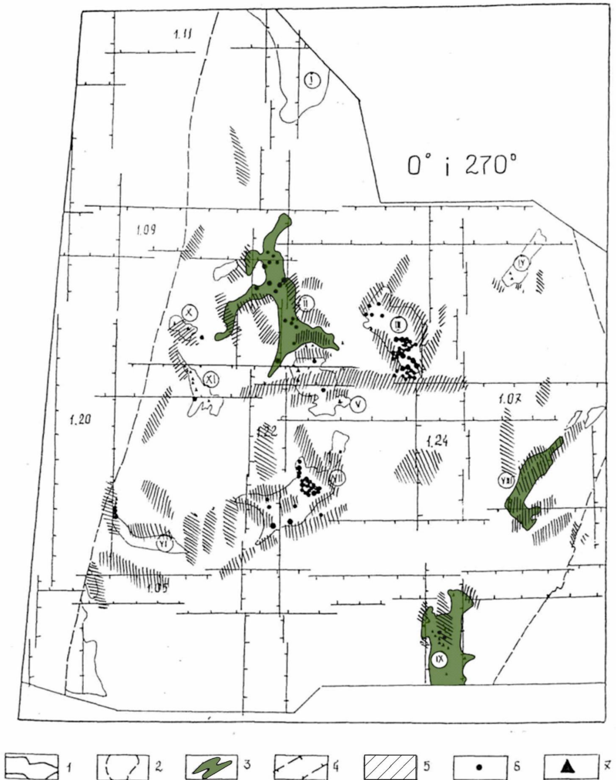
Рисунок 3.33 – Розташування золоторудних проявів, ділянок метосоматозу та зеленокам'яних структур відносно системи розломів з азимутами простягання 0° і 270° (Умовні позначення на стор. 92)
