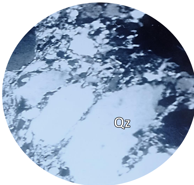
Рисунок 3.14— Орієнтування сплюснених уламків кварцу уздовж сланцюватості в метаконгломератобрекчії тимошівської товщі.
