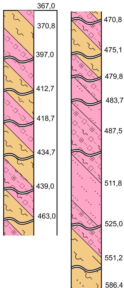
Рисунок 3.15 – Літологічна колонка по свердловині №267 Переверзівської світи (тимошівської товщі). Умовні позначення на рис. рис.3.18.
