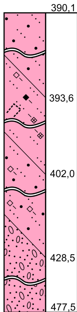
Рисунок 3.16 - Геологічна колонка по свердловині №313.
