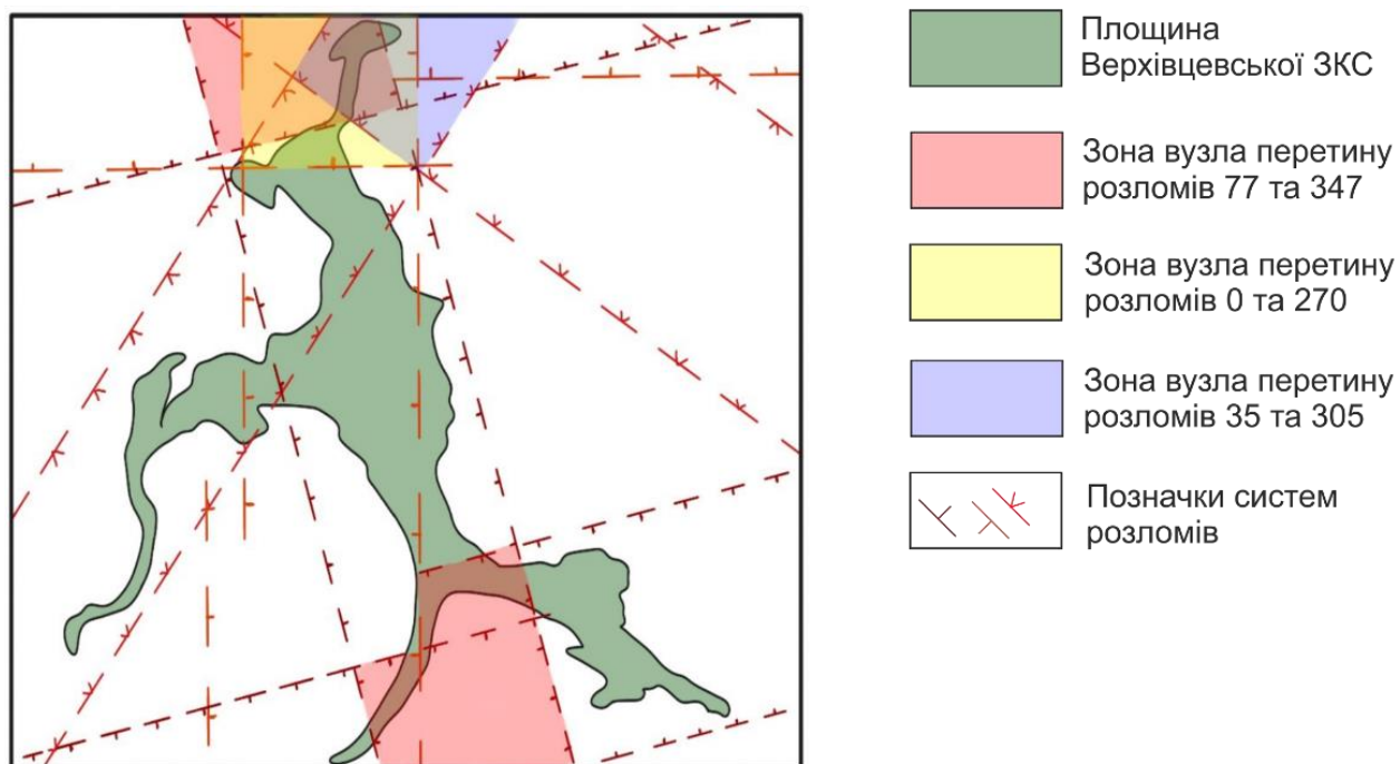
Рисунок 3.32 – Розташування Верхівцевської ЗКС у вузлах перетину систем глибинних розломів
