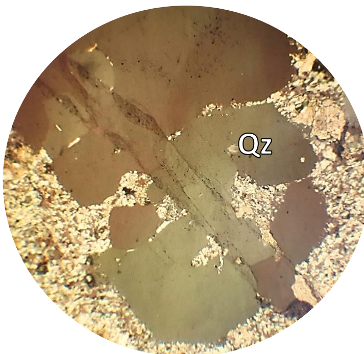
Рис.4.6 - Агрегати кварцу, що кородуються кварц-серицитовими агрегатами з флюїдальною мікротекстурою в цементі метаконгломератобрекчії.
